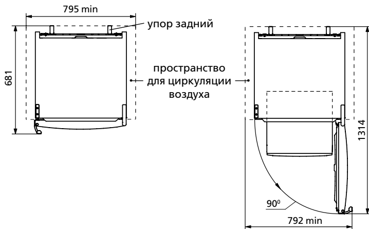
Рисунок 2 — Холодильник (вид сверху)
