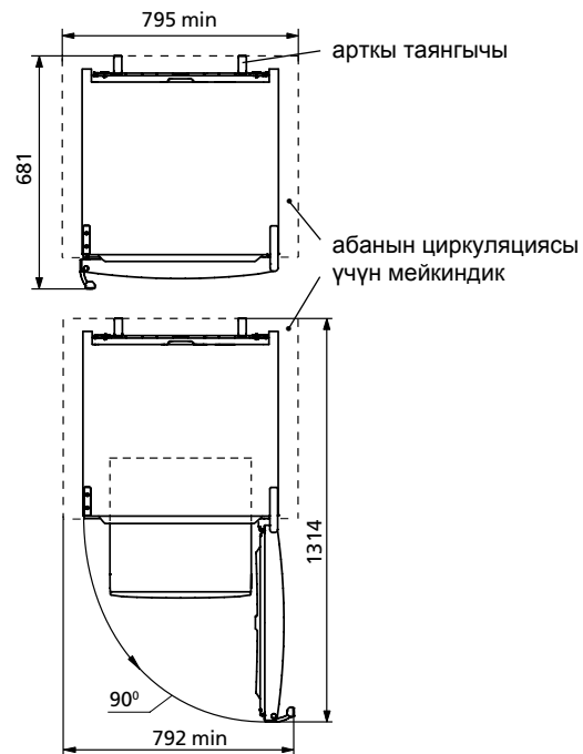
2-сүрөт — Муздаткыч (жогору жагынан көрүнгөн көрүнүшү)
