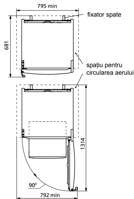
Imagine 2 — Frigider (vedere de sus)
