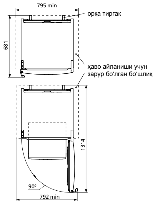
2-расм — Совутқич (уст қисми билан кўриниши)
