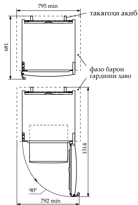
Расми 2 – Яхдон (намуди он аз боло)
