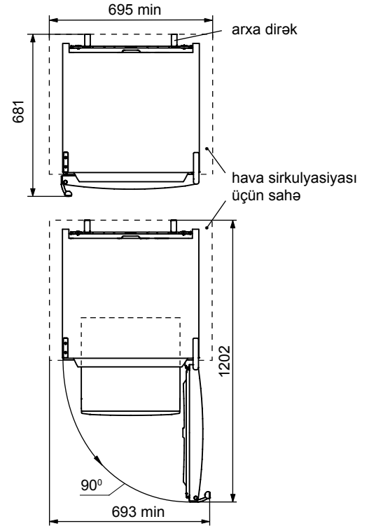
Şəkil 2 – Soyuducu (yuxarıdan görüntüsü)
