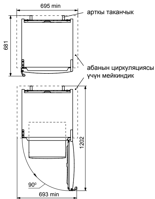
2-сүрөт – Муздаткыч (үстүнөн караганда)
