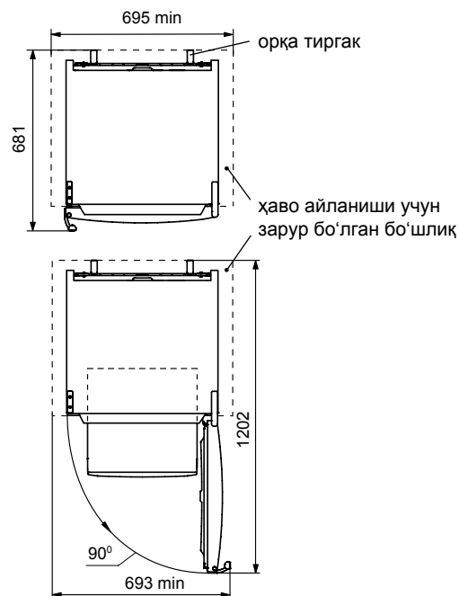
2-расм – Совуткич (юқоридан кўриниши)
