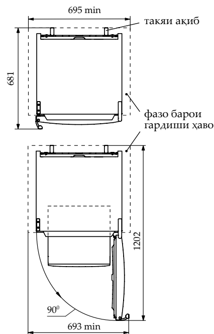
Расми 2 – Яхдон (намои болоӣ)
