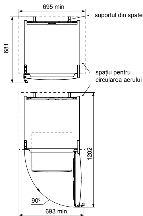
Figura 2 – Frigiderul (privire de sus)
