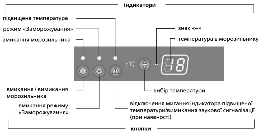
Рисунок 3 – Блок керування
