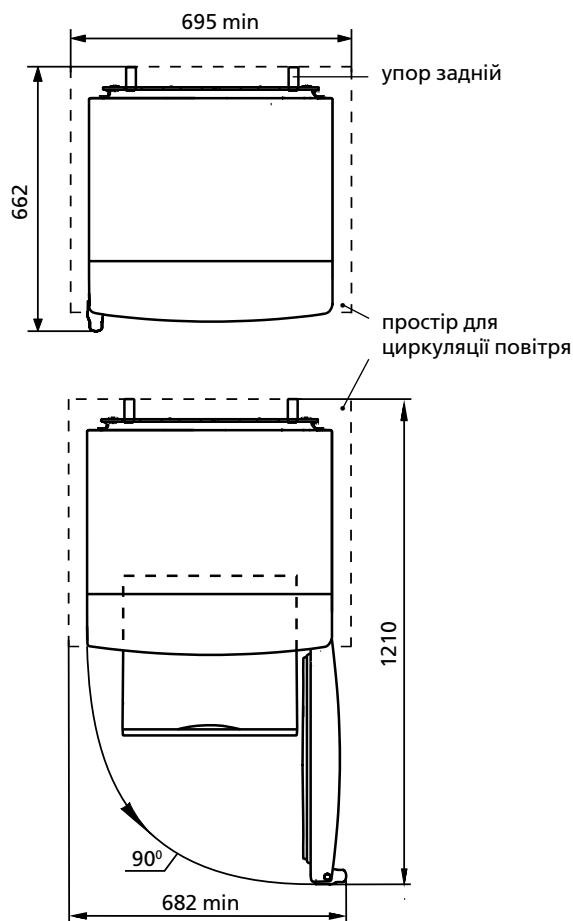
Рисунок 2 – Морозильник (вид зверху)
