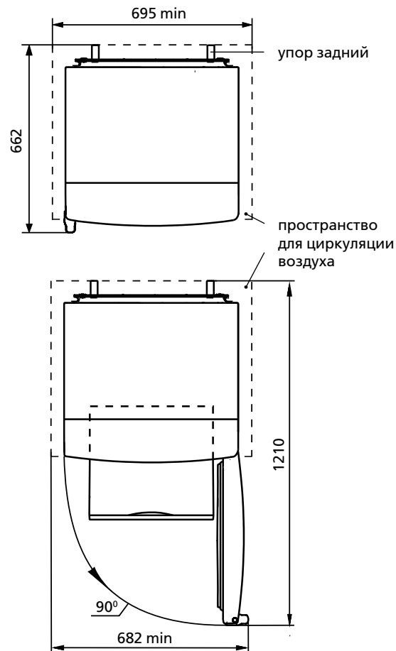
Рисунок 2 – Морозильник (вид сверху)
