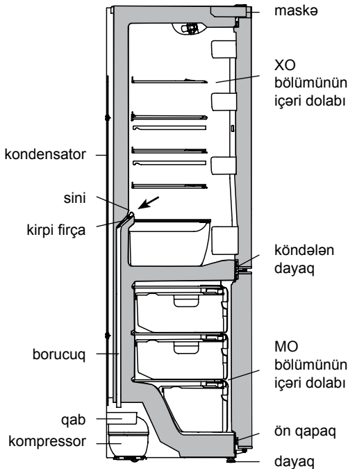
Rəsim 6 – XO bölümünün ərmiş axıntı sularının tökülmesi sxemi
